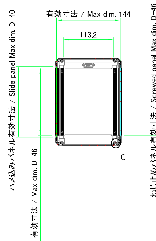
C : フレーム拡大図 / Frame cross-section
