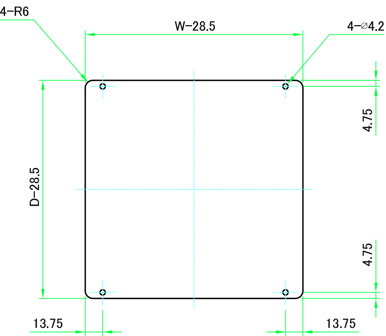
パネル裏面 / Panel Backside
